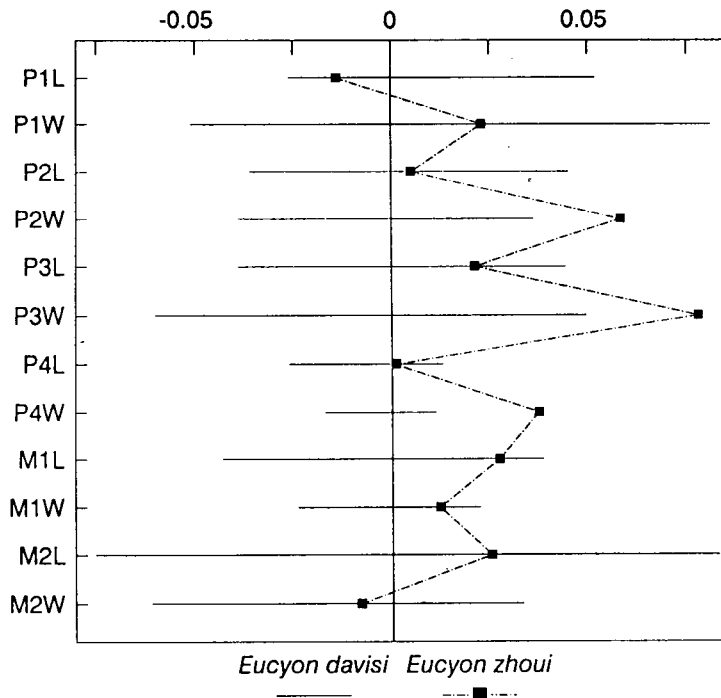
图3 Eucyon 两个种的牙齿对数比率图(Simpson 1941)，数据取自表1 E. davis (对比基)，峡口材料，七个个体，横线为观测数据； E. zhoui ，五个个体，仅取均数
