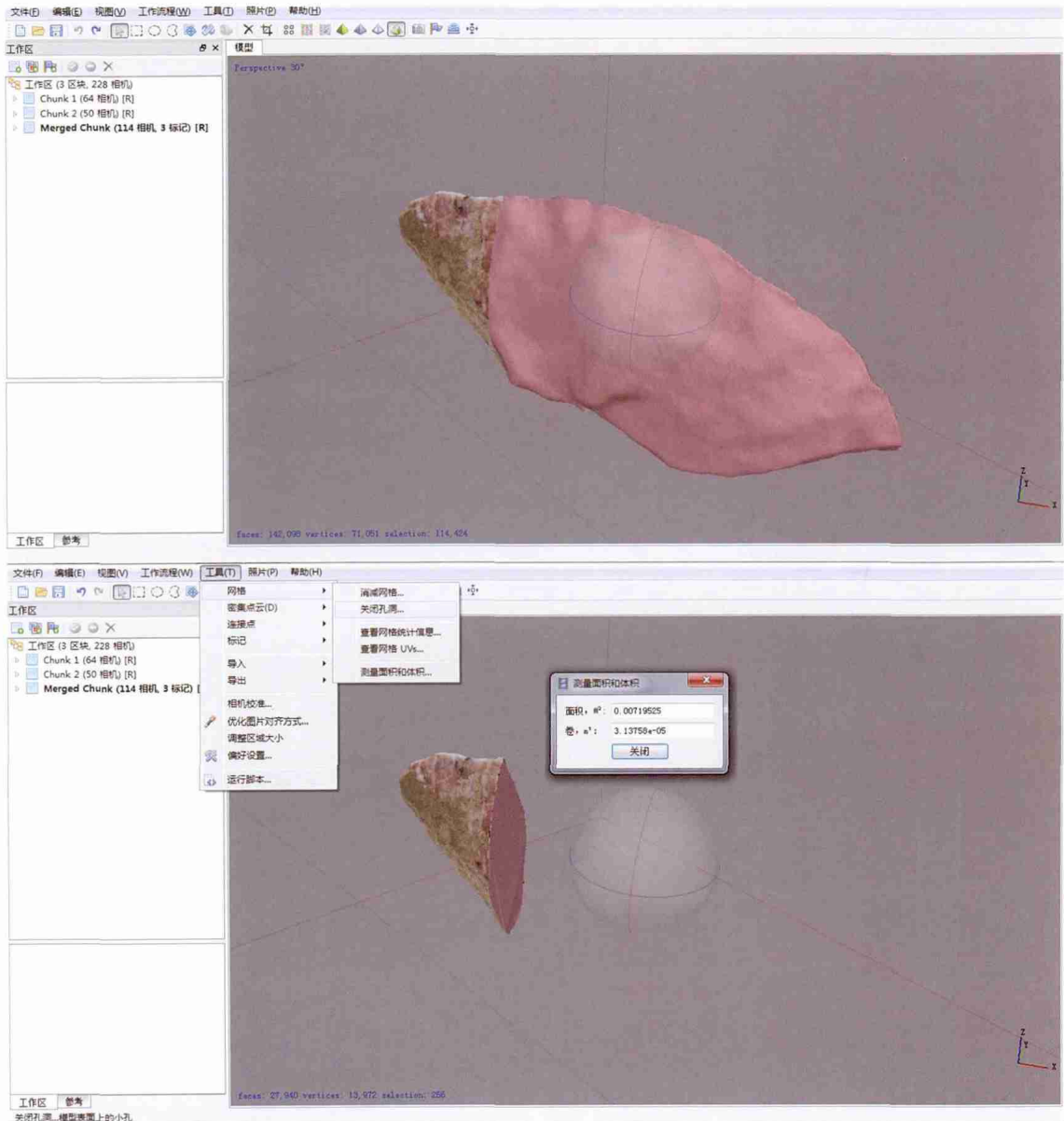
图 5 器物局部体积测量 Fig.5 Volume precise measurement
