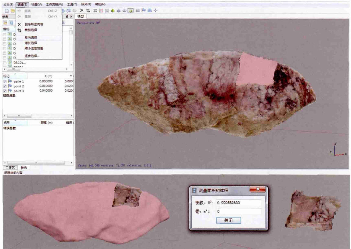
图 6 器物局部表面积测量 Fig.6 Area precise measurement
