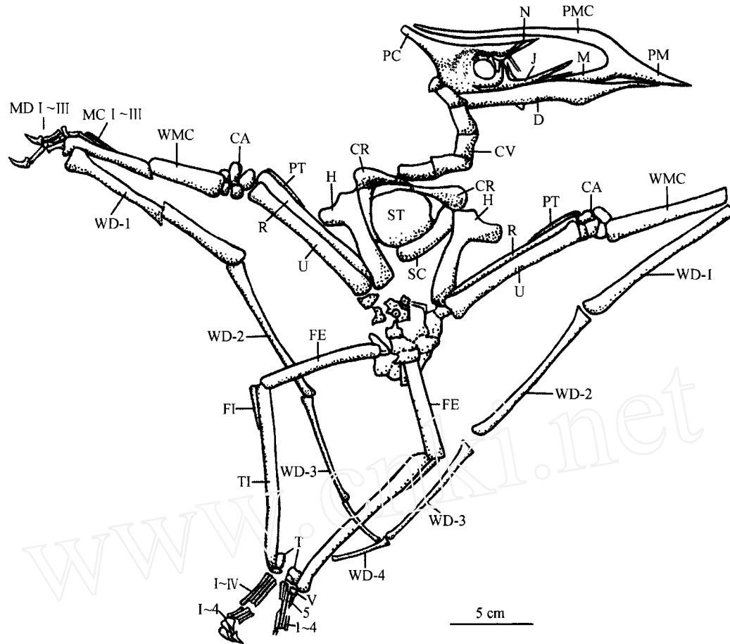
图1 董氏中国翼龙(新属、新种) Sinopterus dongi gen. et sp. nov.正型标本(IVPP V 13363)轮廓图
