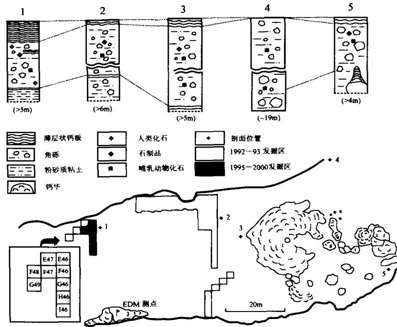
图 1 盘县大洞平面图和沉积剖面图
