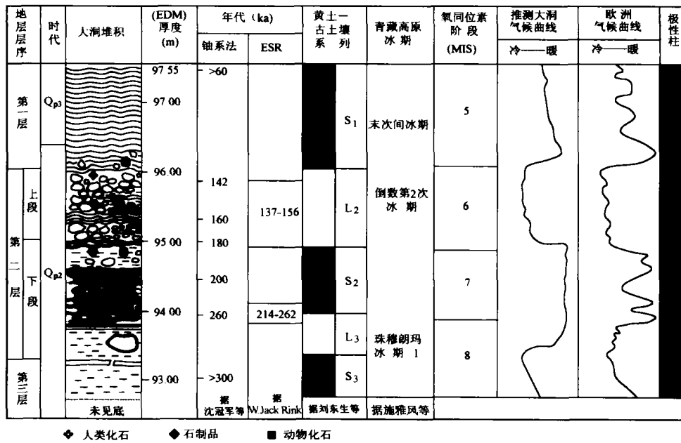
图 2 盘县大洞堆积物的古气候环境对比
