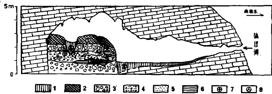
图2 福建清流洞口村狐狸洞人类化石产地剖面示意图
